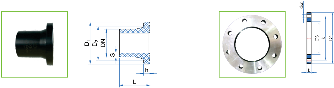
Đầu nối bằng bích và vành bích thép - Stub flange and backing ring
