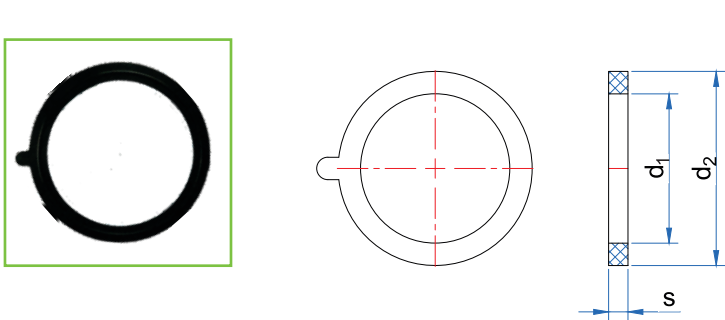
Gioăng bích PE - Gasket for PE flange
